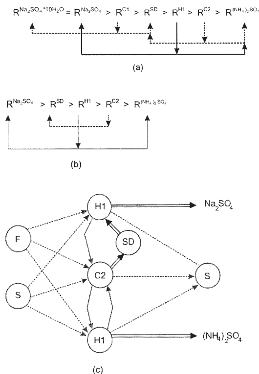
Figure 4. \text{Na}_2\text{SO}_4 + (\text{NH}_4)_2\text{SO}_4 + \text{H}_2\text{O} system.
